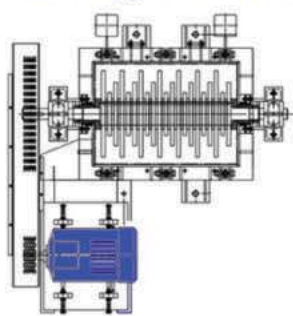
Roots Chopper มัดสับหัวมัน
